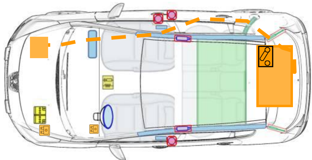
Ni-MH 200 V batterie
